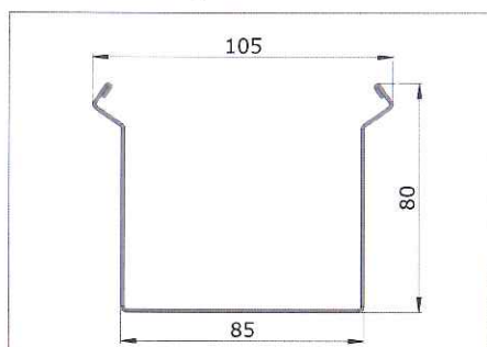
Versteviging bochten
